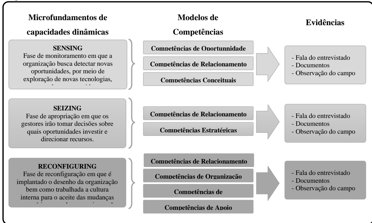
Figura 1 - Modelo Teórico
